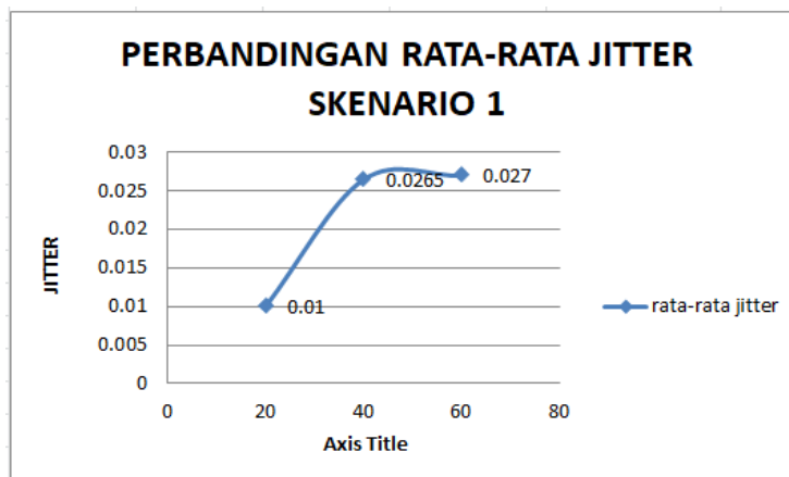
Gambar 6. Grafik rata-rata jitter skenario 1
