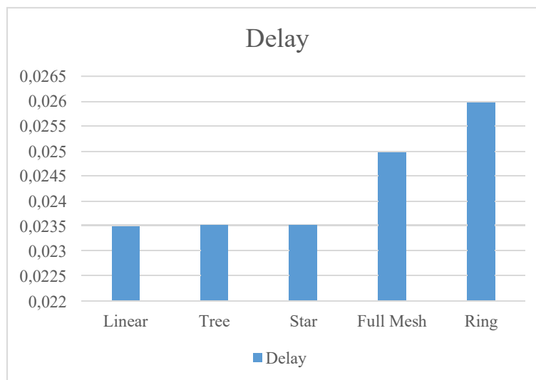
Gambar 8. Perbandingan Delay pada Topologi.
