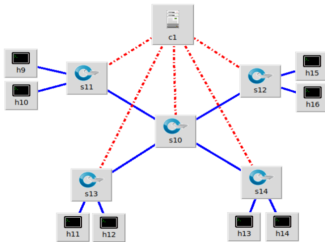
Gambar 5. Topologi Star
